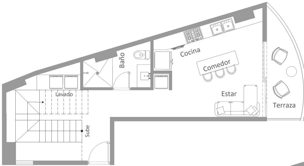
PLANTA BAJA
