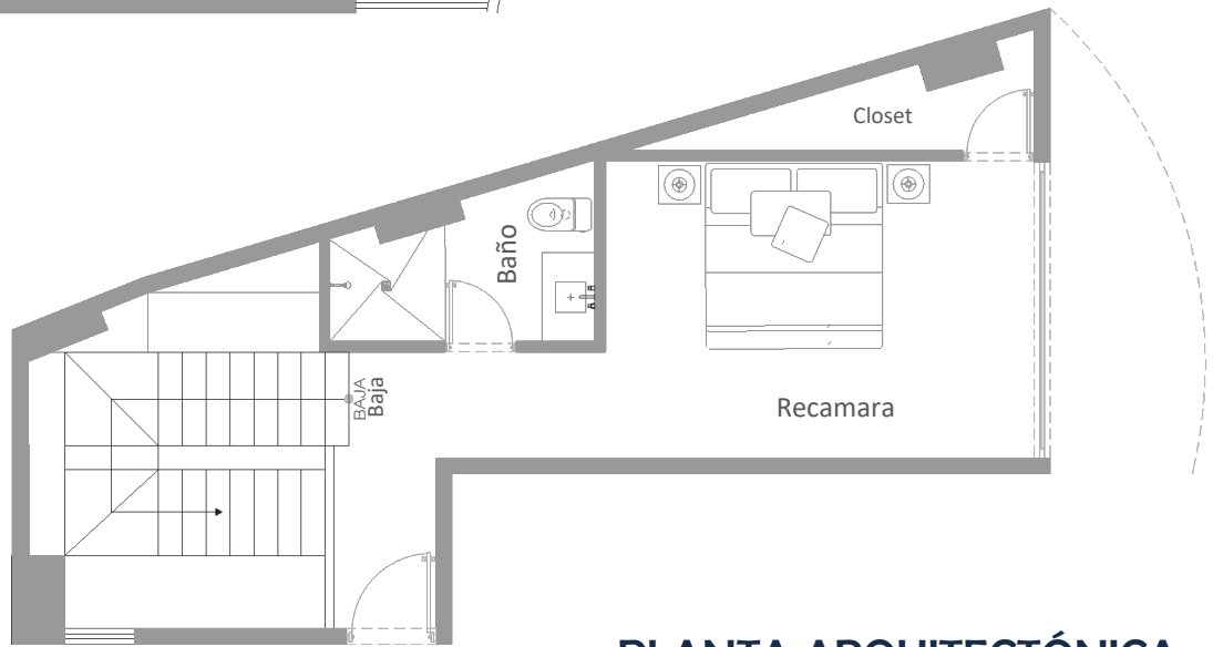
PLANTA ALTA
